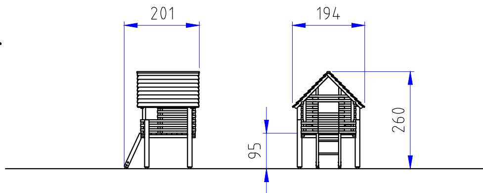
903312100L Pfahlhaus
